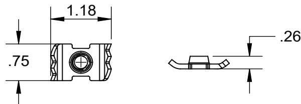
3) T-Nut, Sheet Metal
